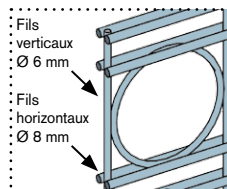
FRISE DÉCORATIVE Fils acier et dimensions ronds
